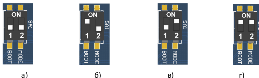
Рисунок 13. Переключатель SA1 :
